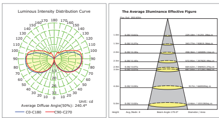
6W GLOW BAR 38204-012
