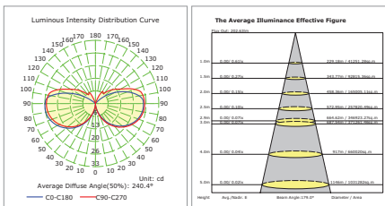
6W GLOW BAR 38204-012
