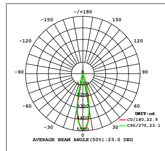
14W - 3500K - 20°
