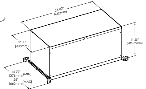
AIRTIGHT IC BOX 44366-018 IC BOX 44365-011
